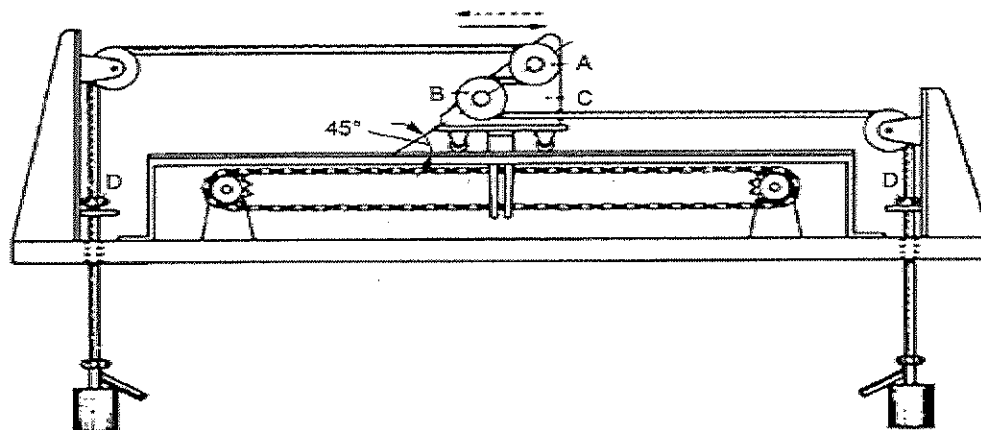
A, B – ролики; C – каретка; D – удерживающий зажим
