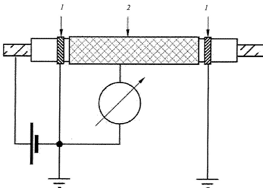
1 – защитный электрод (защитный проволоочный бандаж); 2 – экранный электрод (электропроводящий слой, поверх которого наложена металлическая оплетка или металлическая лента)
