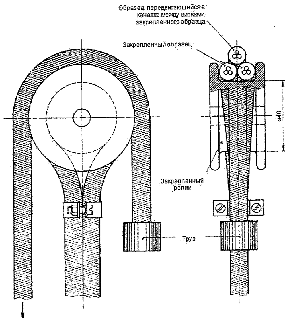
Рисунок 5 – Устройство для испытания на износостойкость
